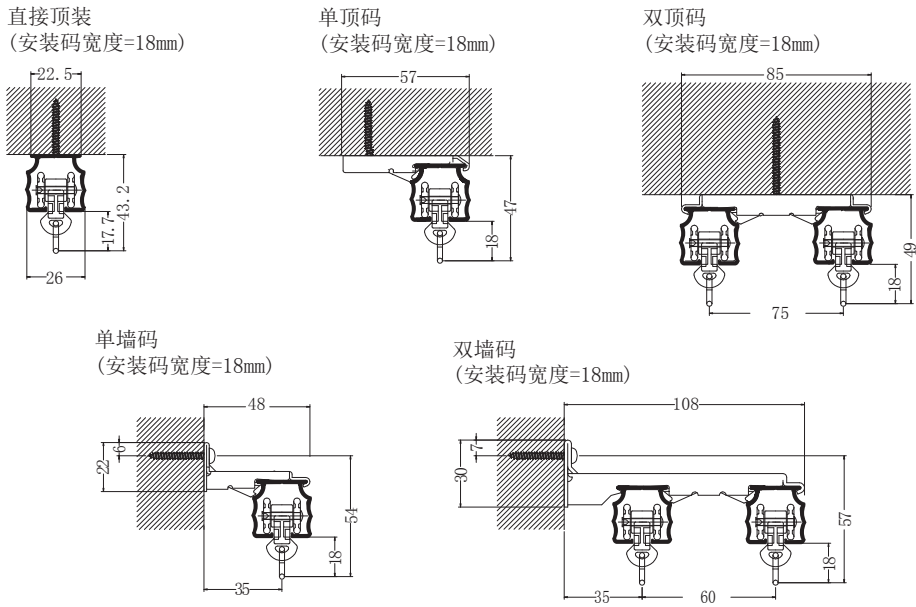
安装示意图 (单位:mm)
