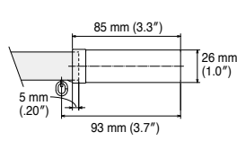
End Cap B
